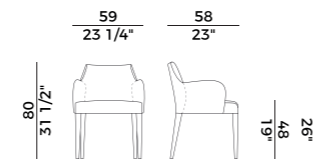
772/PI poltrona \ armchair
